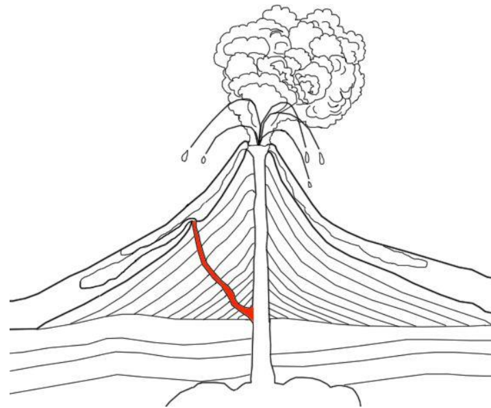
cheminée secondaire
