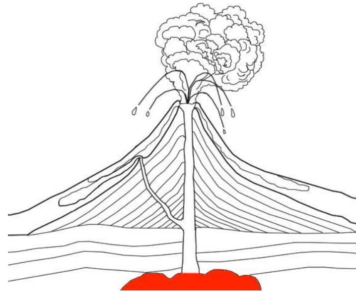
chambre magmatique
