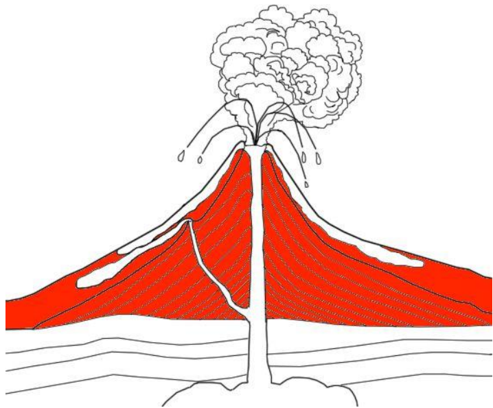
cône volcanique
