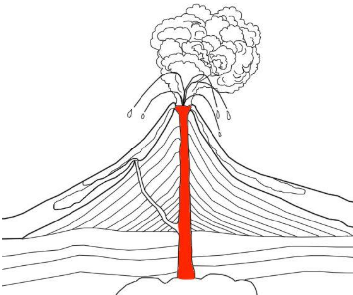
cheminée principale
