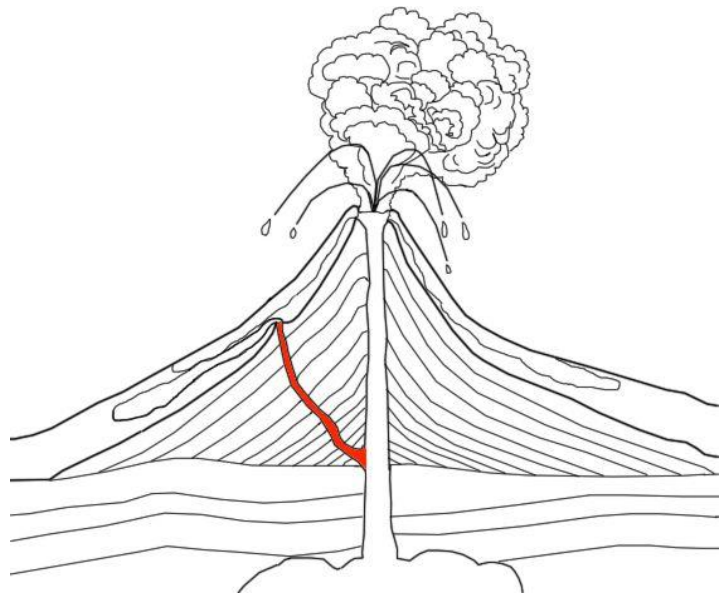
cheminée secondaire
