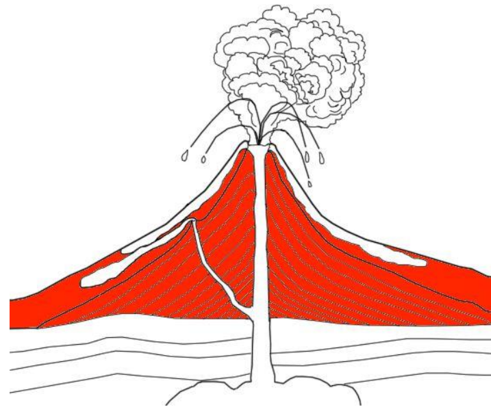
cône volcanique
