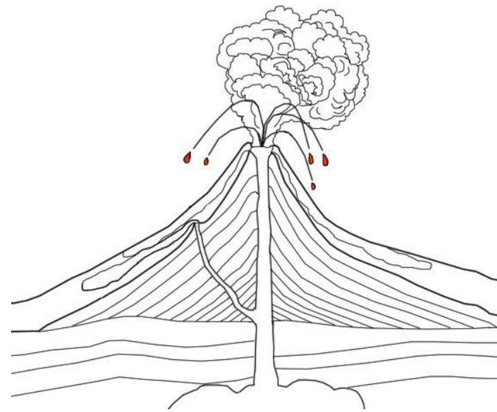
bombes volcaniques
